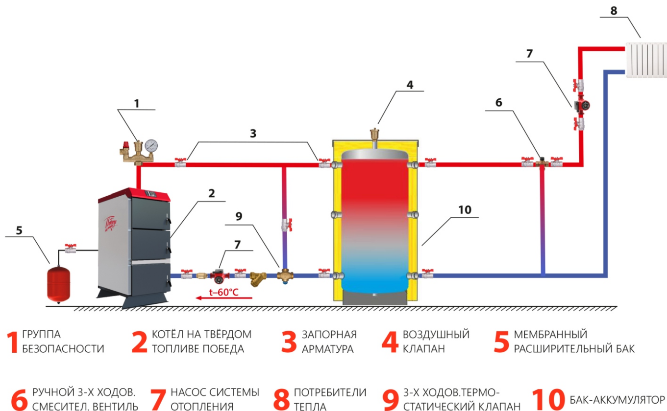
Рисунок 3 - Подключение с баком-аккумулятором
